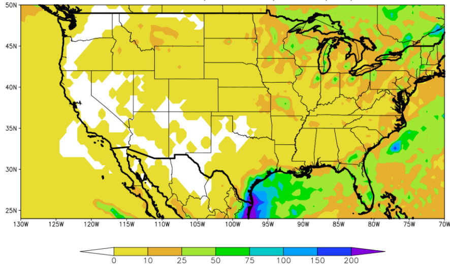
PERSPECTIVA SEMANAL 9 al 15 de Septiembre de 2021 PRECIPITACION (Escala mm) NIEVE (Gris)
