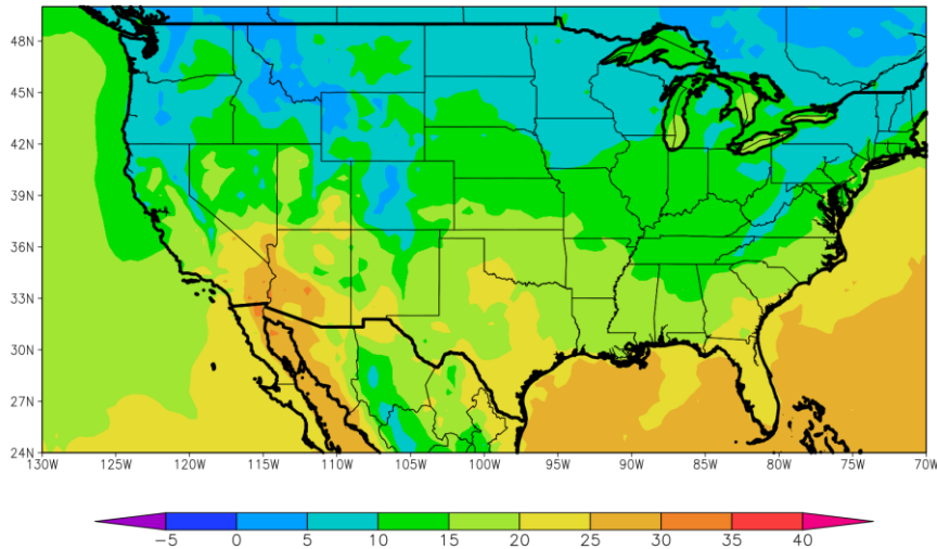
PERSPECTIVA SEMANAL 9 al 15 de Septiembre de 2021 TEMPERATURA MINIMA(Grados Cent.)
