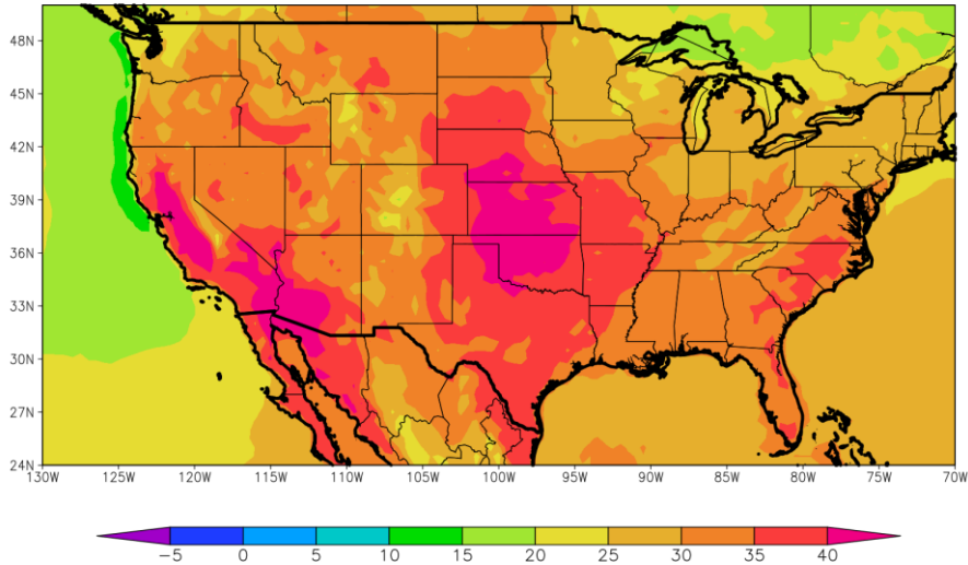
PERSPECTIVA SEMANAL 9 al 15 de Septiembre de 2021 TEMPERATURA MAXIMA(Grados Cent.)
