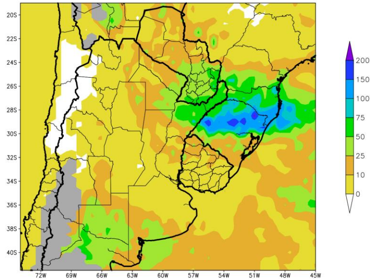
PERSPECTIVA SEMANAL 16 al 22 de Septiembre de 2021 PRECIPITACION (Escala mm) NIEVE (Gris)
